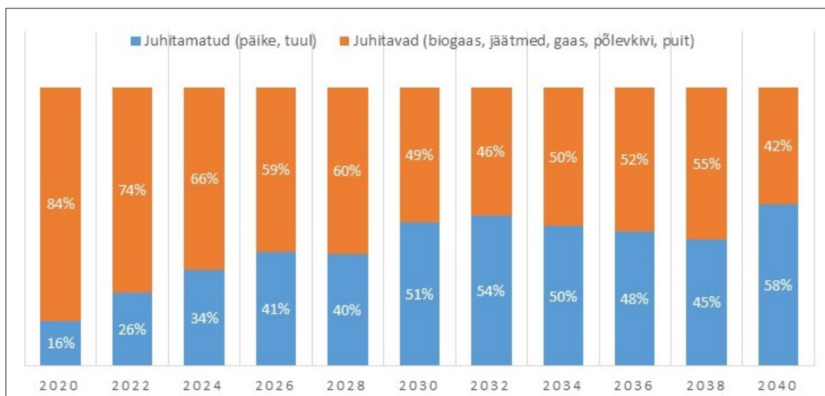
Joonis 6. Prognoos kontrollitavate ja muutlike elektrilike võimsuste osakaalu kohta Eesti elektritootmises, lähtudes „Eesti riiklikust energia- ja kliimakavast aastani 2030“
