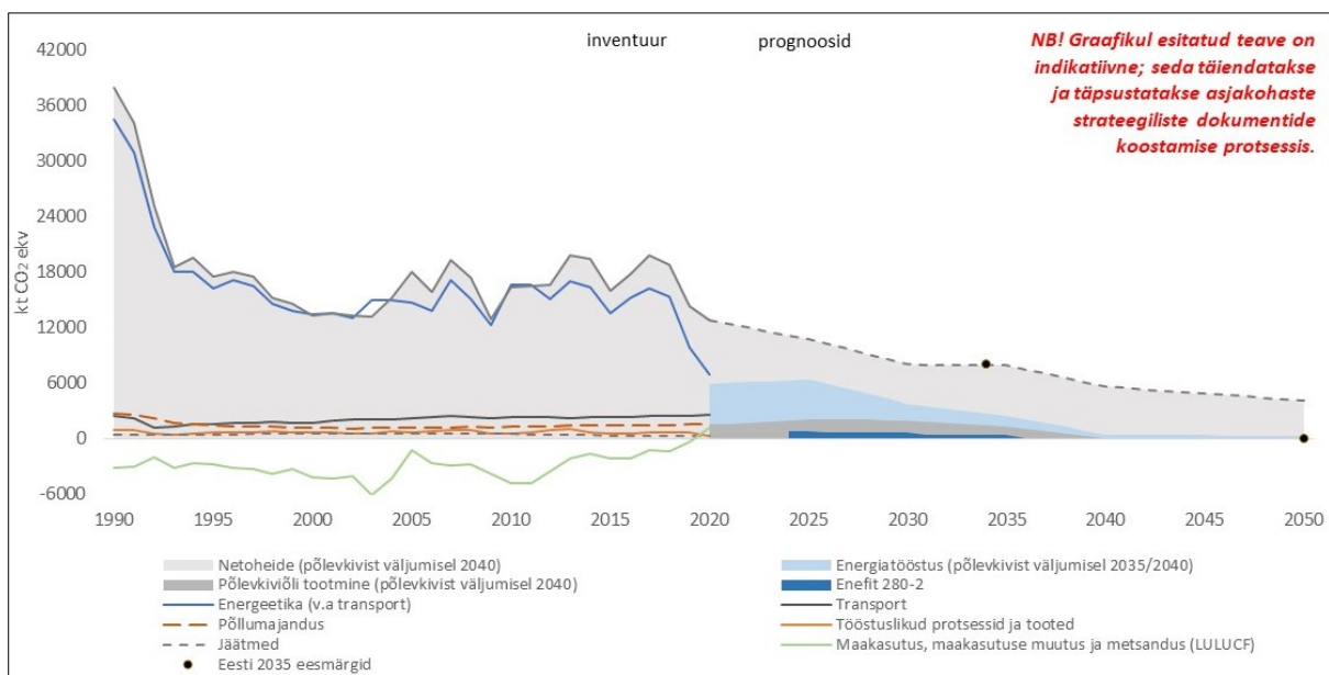
Joonis 2. Eesti KHG heitkogused perioodil 1990–2020 (kt CO 2 ekv) ning illustratiivne teekond kliimaneutraalsuse saavutamiseni energeetikatööstuse sektoris koos selle mõjuga teistele sektoritele. Graafik kirjeldab stsenaariumi, mis põhineb Eesti valitsuse eesmärgil lõpetada elektri tootmine põlevkivist hiljemalt aastaks 2035 ning loobuda pk kasutamisest energeetikas tervikuna hiljemalt aastaks 2040 (nn stsenaarium SEN2). Graafik on indikatiivne ning on koostatud värseima kättesaadava teabe (sh otse põlevkivisektori tuumikettevõtelt pärineva teabe) põhjal. Lähteandmed täpsustuvad asjakohaste strateegiliste dokumentide koostamise protsessis. Graafikul on eraldi välja toodud Eesti Energia poolt rajatava keemiatehase (Enefit 280-2) mõju Eesti KHG heitele.
